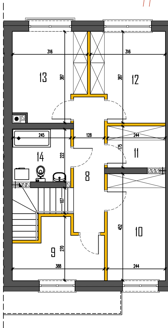
RZUT PIĘTRA
